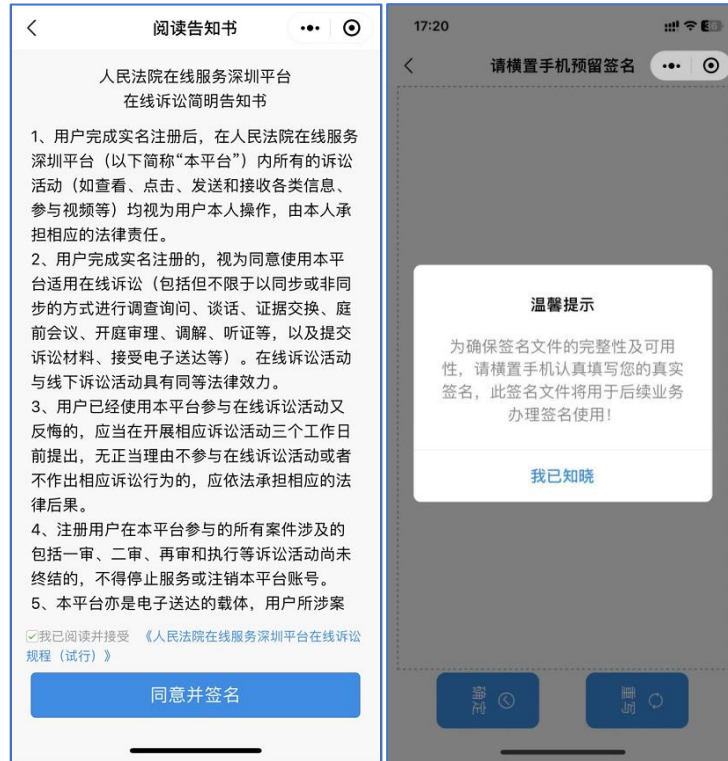
图 1.1-5 在线签名
