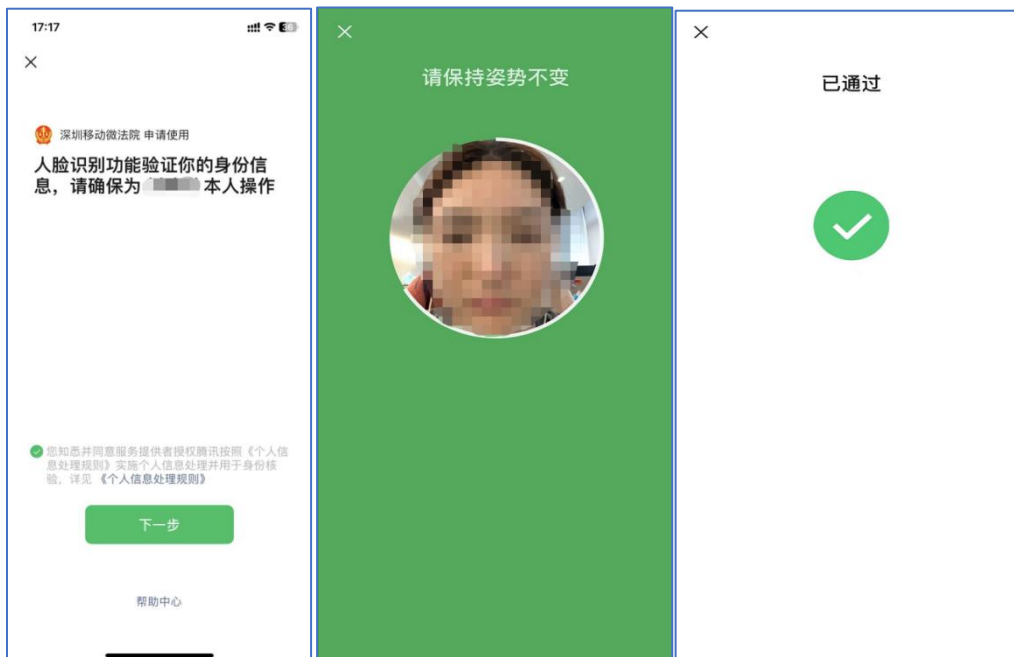
图 1.1-4 人脸识别
