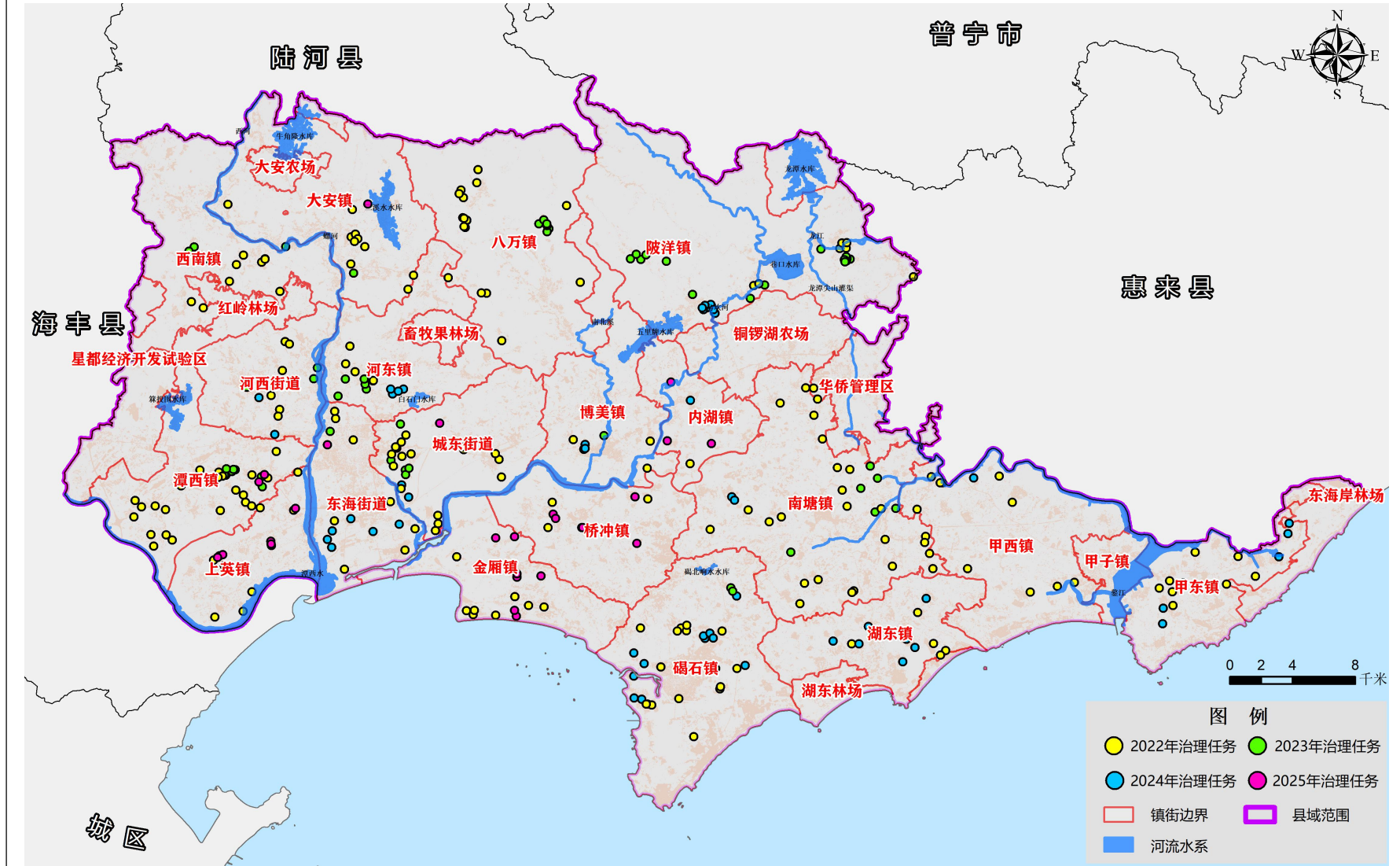
陆丰市农村生活污水治理时序规划图
